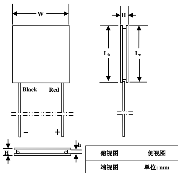
图 6. 密封ATE1-241的机械尺寸
