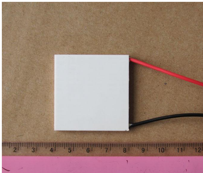
图 1 ATE1-241 的实体照片
