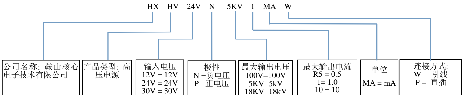
图 10、HXHV24VN5KV1MAW 的命名说明
